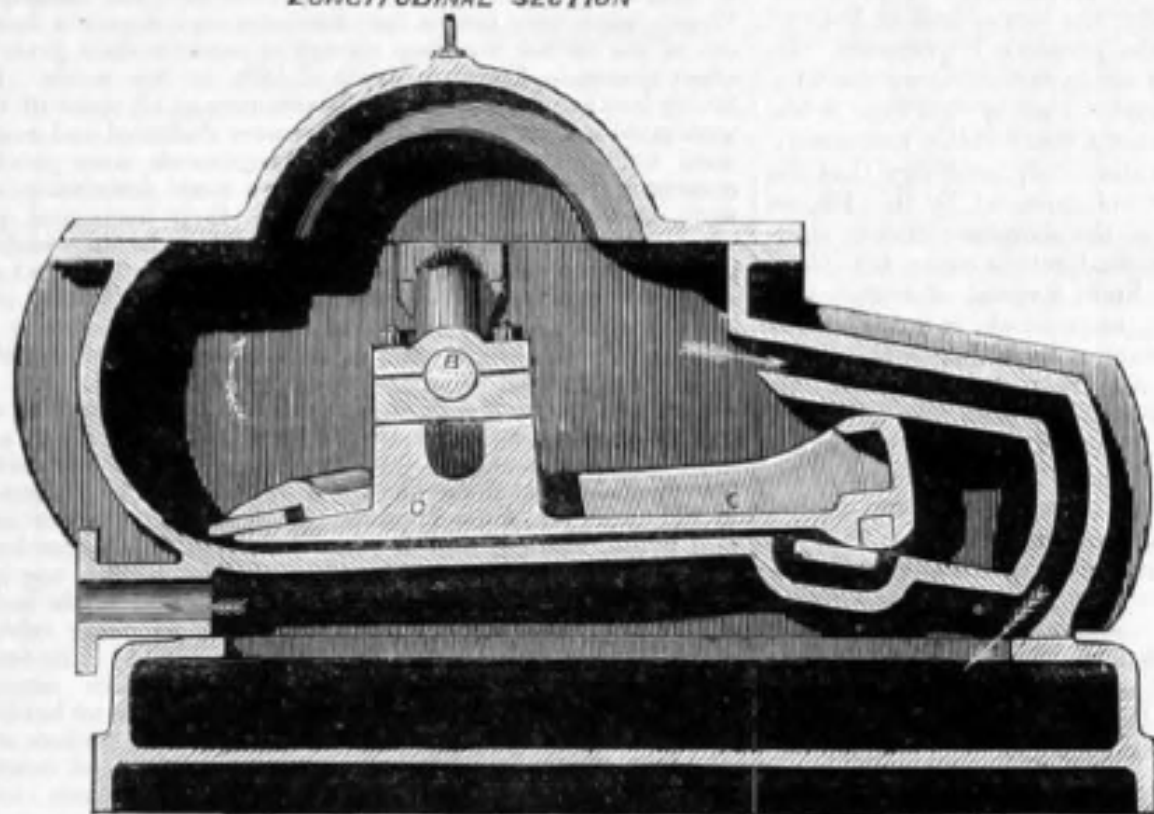
LONGITUDINAL SECTION
